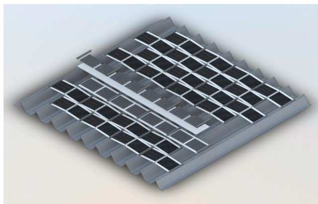
シート工法
